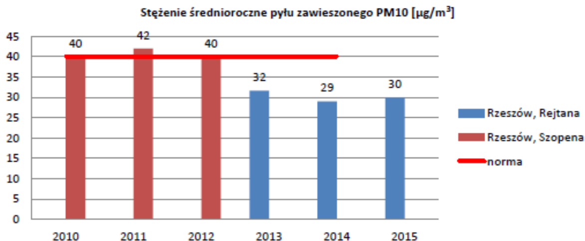
Rysunek 4. Wyniki pomiarów stężeń średniorocznych pyłu PM10 na stanowiskach pomiarowych w Rzeszowie w latach 2010-2015 (Źródło: Aktualizacja Programu ochrony powietrza dla strefy miasto Rzeszów – z uwagi na stwierdzone przekroczenia poziomu dopuszczalnego pyłu zawieszonego PM10 i poziomu dopuszczalnego pyłu zawieszonego PM2,5 wraz z rozszerzeniem związanym z osiągnięciem krajowego celu redukcji narażenia i z uwzględnieniem poziomu docelowego benzo(a)pirenu oraz z Planem Działań Krótkoterminowych” Autor: ATMOTERM S.A., Rzeszów, 2016 r.).
